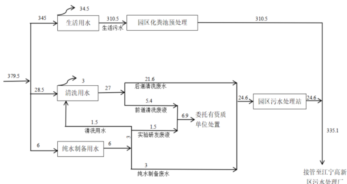
图 2-1 全厂水平衡图（单位： \text{m}^3/\text{a} ）
